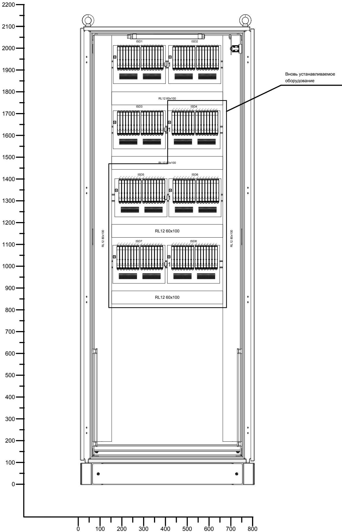
Вид сзади без дверей
